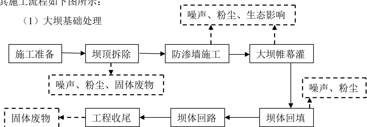
图 4-1 大坝基础处理工艺流程图
