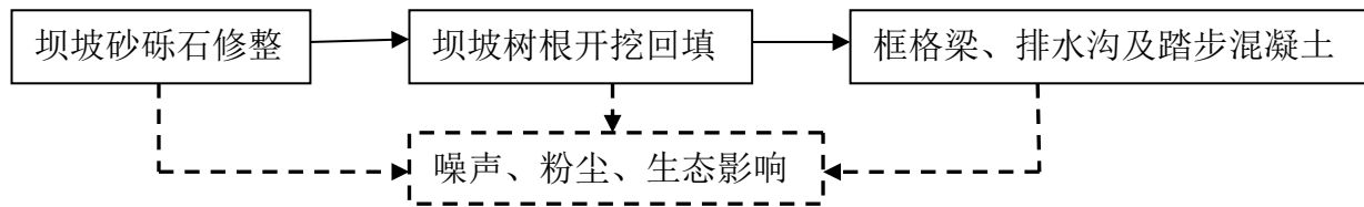
图 4-3 护坡加固施工工艺流程图
